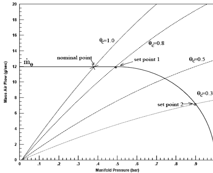
Gambar 3.3 Trajectories dari air flow untuk \theta = 10 yang masuk ke manifold ( m_{\theta}^{\text{U}} )
